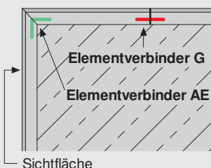
bei Balkonabschaler
